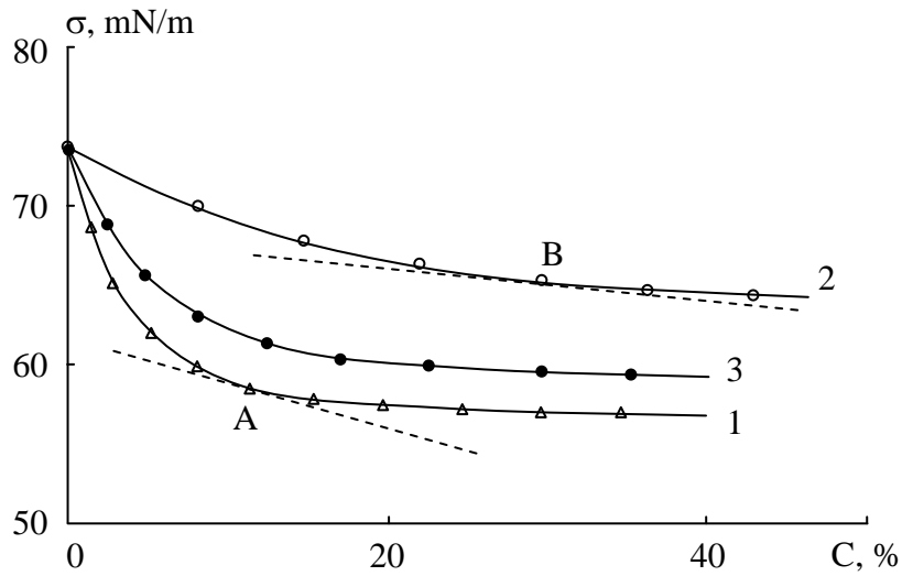
Şək. Səthi gərilmə əmsalının məhlulun konsentrasiyasından asılılığı. 1-PEQ-su, 2-qliserin-su, 3-PEQ-qliserin-su məhlulu (PEQ-in konsentrasiyası ümumi məhlulun 20%-ni təşkil etməklə).
